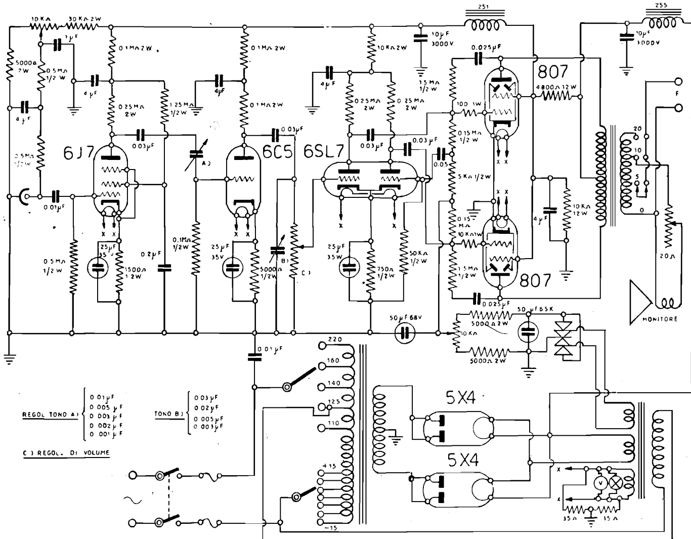
OFFICINE A. PREVOST - Impianto da cinema sonoro di grande potenza, da 40 watt, mod. 401. Ciascuno dei due controlli di tono indicati con i condensatori fissi, come nello schema di fig. 782.
